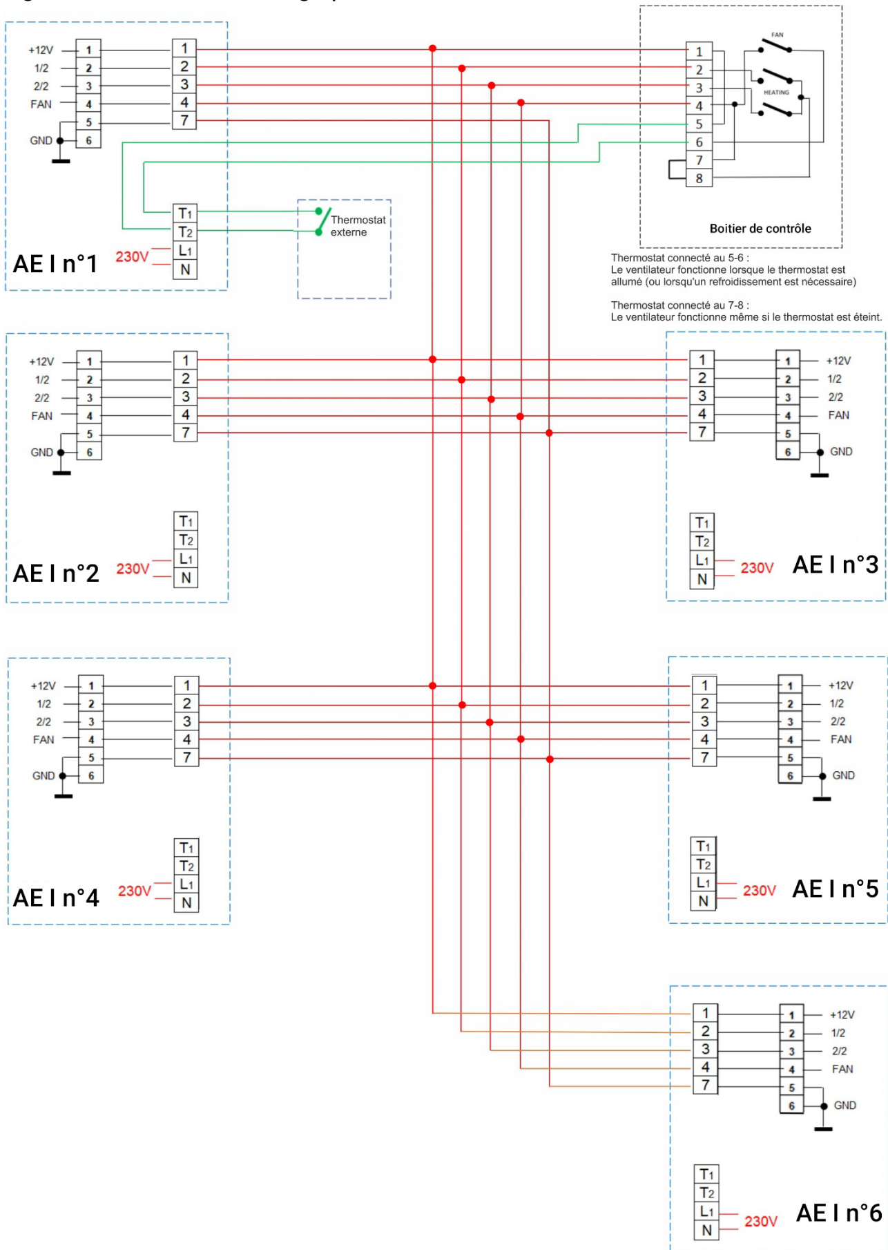
Figure 6. Schéma de câblage pour une installation de 2 à 6 aérothermes (modèle 3,3 kW)
