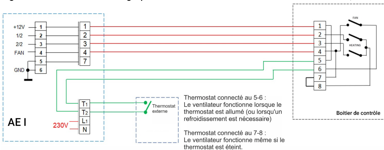
Figure 5. Schéma de câblage pour une installation d'un seul l'aérotherme (modèle 3,3 kW)
